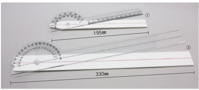
Goniometer
