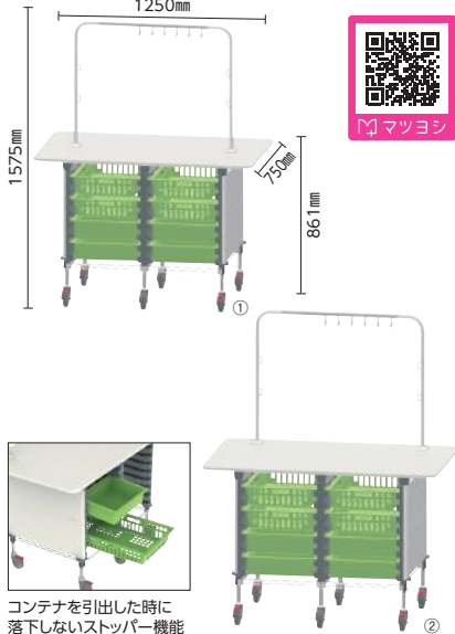
コンテナを引出した時に落下しないストッパー機能
